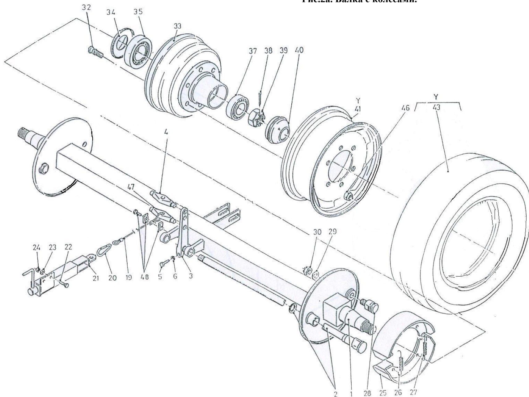
Рис.2а. Балка с колесами.
