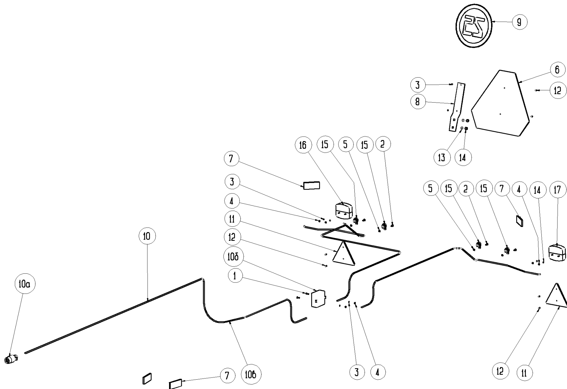
Рис.9. Световая сигнализация
