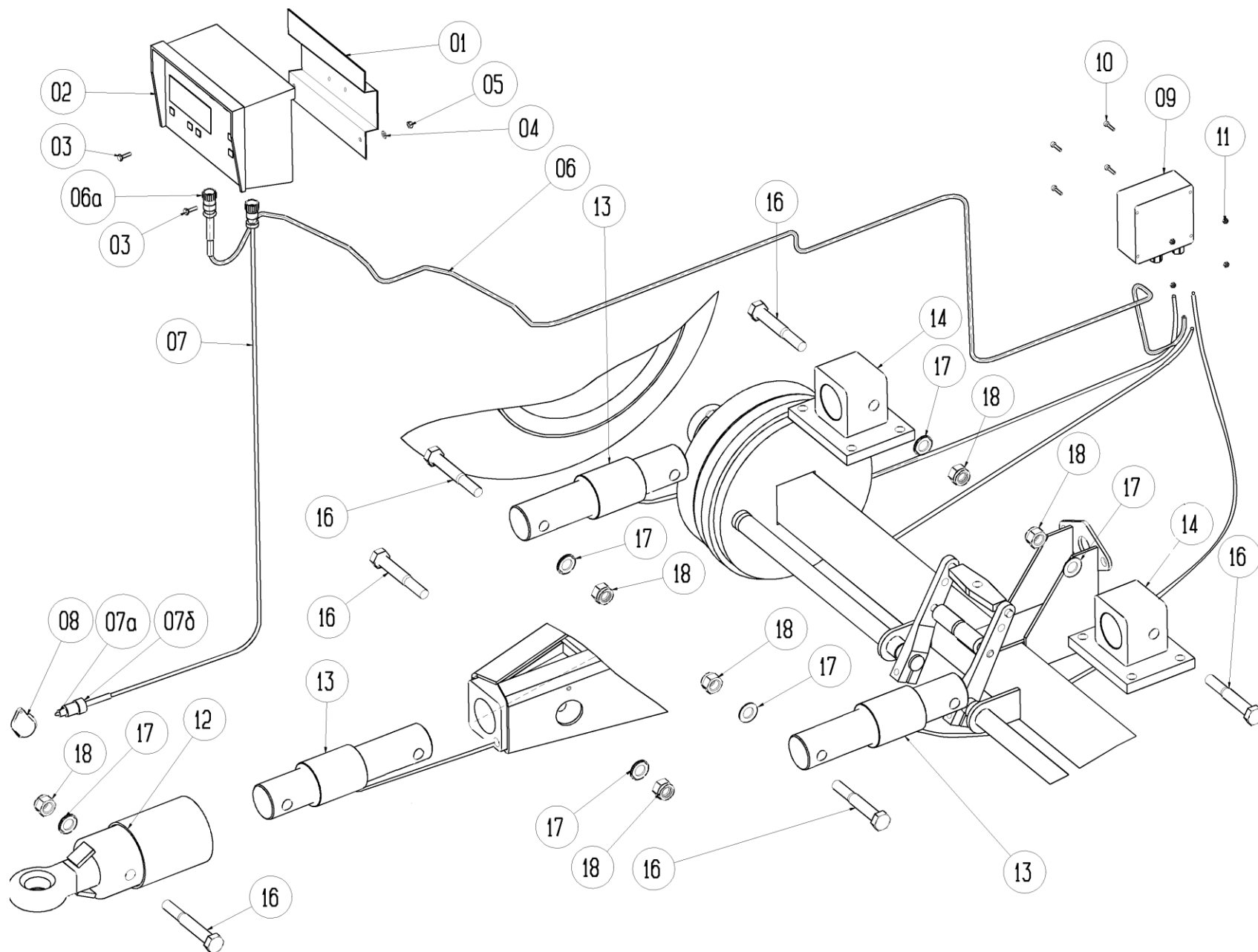
Рис.7. Электронное взвешивающее устройство
