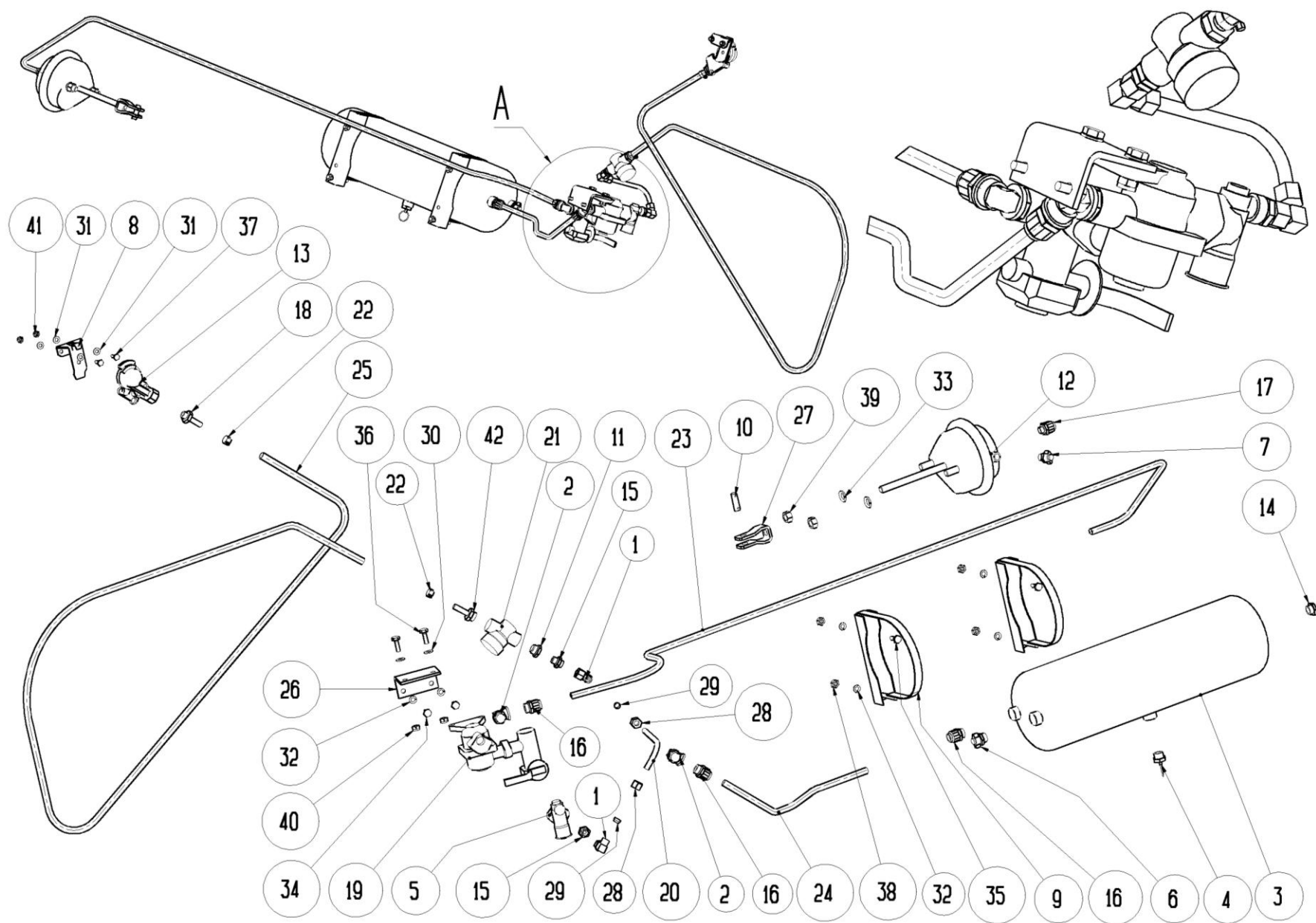
Рис.8. Пневматическая тормозная система
